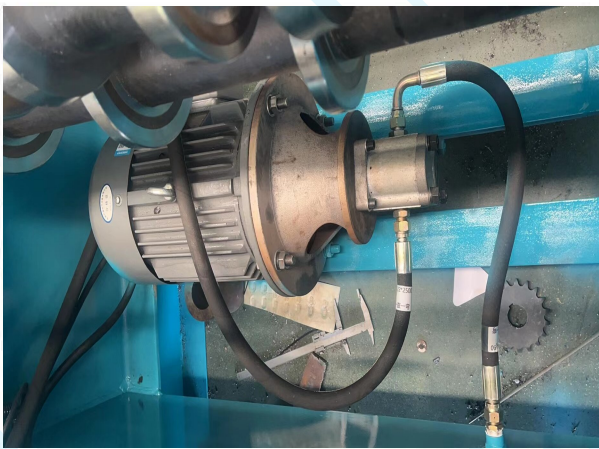
Motor
