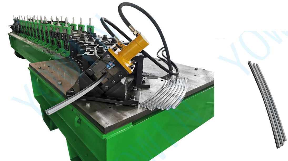
德国宝马玻璃升降器成型机
