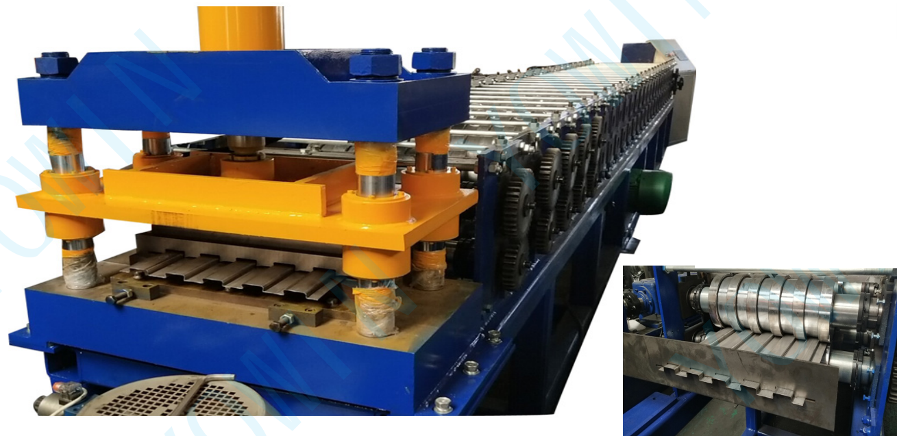
火车车厢版成型机
